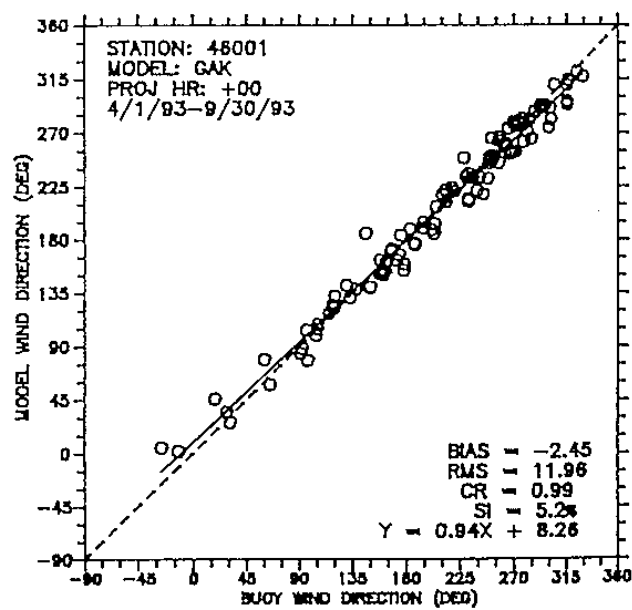
圖 4、GAK 模式的初始 (+00) 波高、風速和風向與實測 值的比較。
