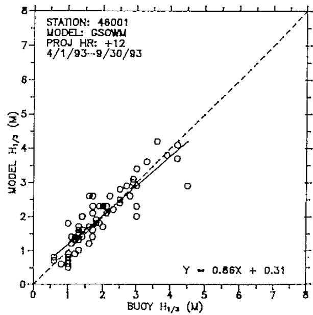
圖 1a、作業化模式 GAK, NOW 和 GSOWM 的預報波高和實測值的比較, (a) +12 時預報。
