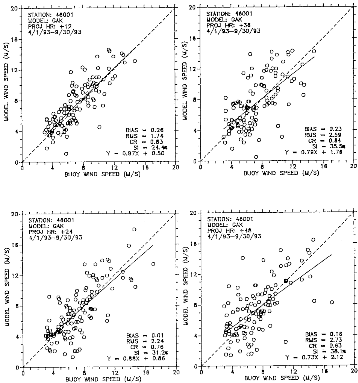
圖 3a、模式預報風場與實測值的比較，(a) 風速；
