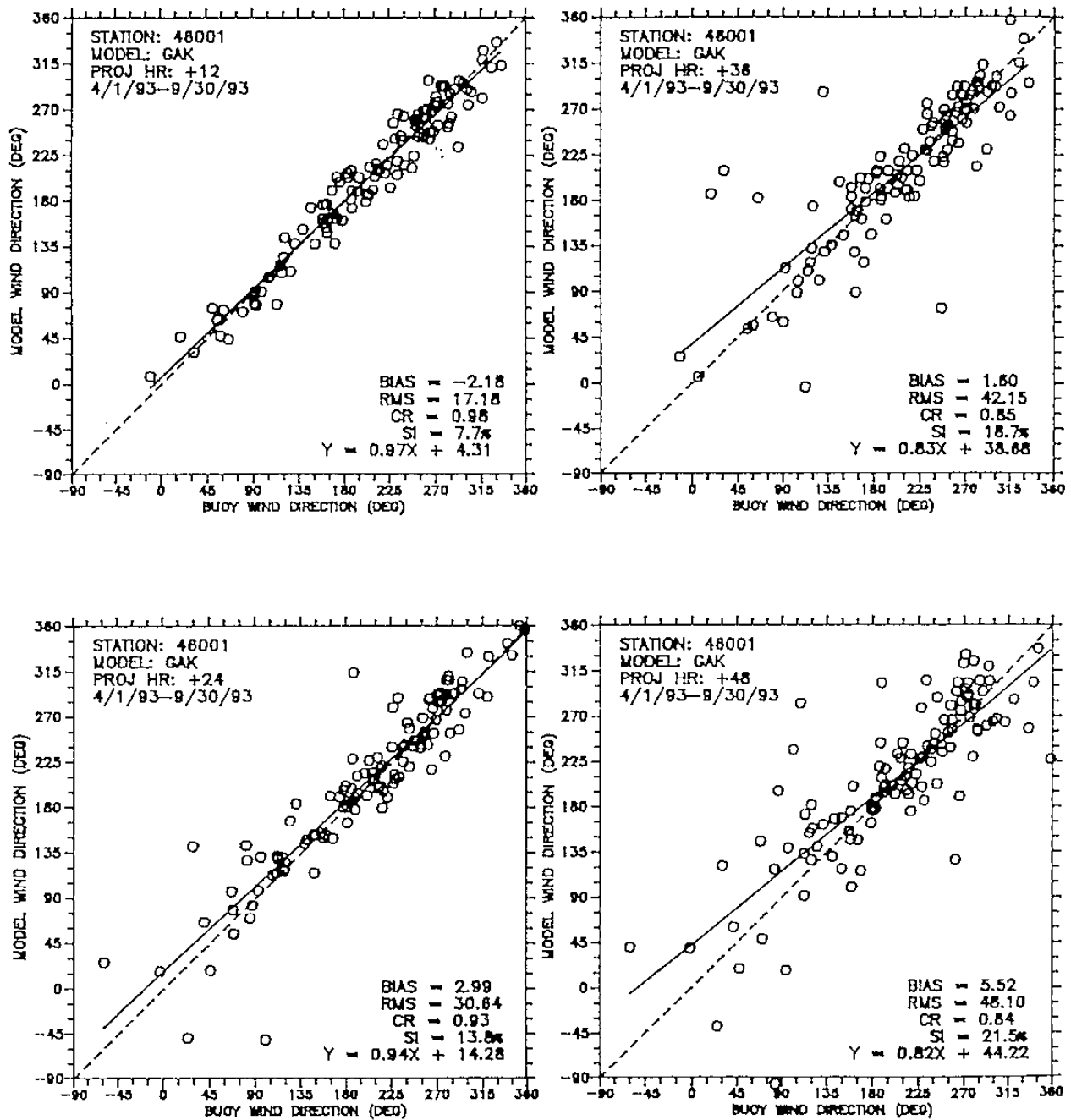
圖 3b、模式預報風場與實測值的比較， (b) 風向。
