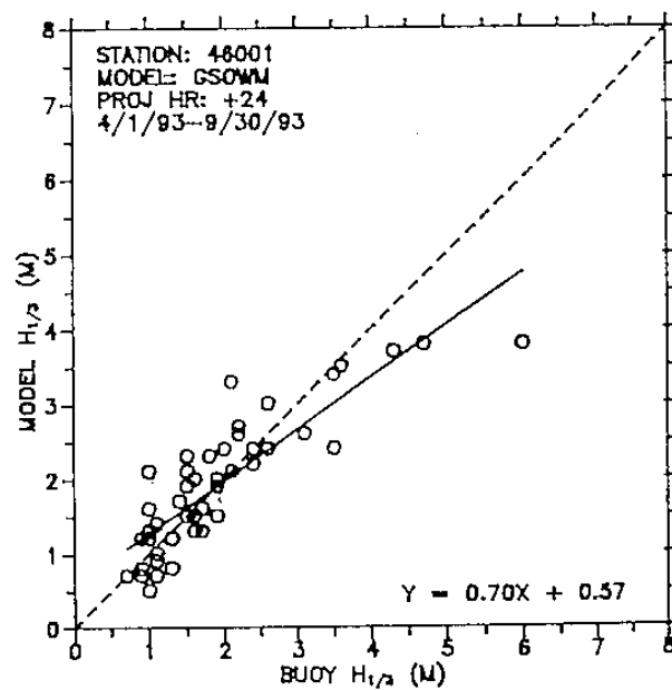
圖 1b- 作業化模式 GAK, NOW 和 GSOWM 的預報波高和實測值的比較 (b) +24 時預報
